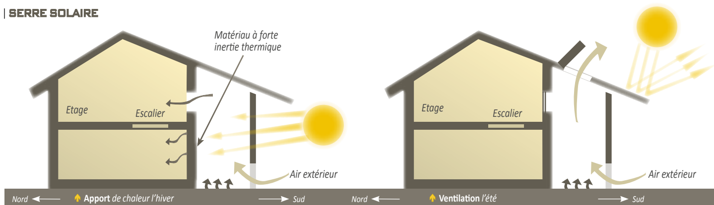
👉 Serre solaire, Stéphanie Etienne, Architecte
